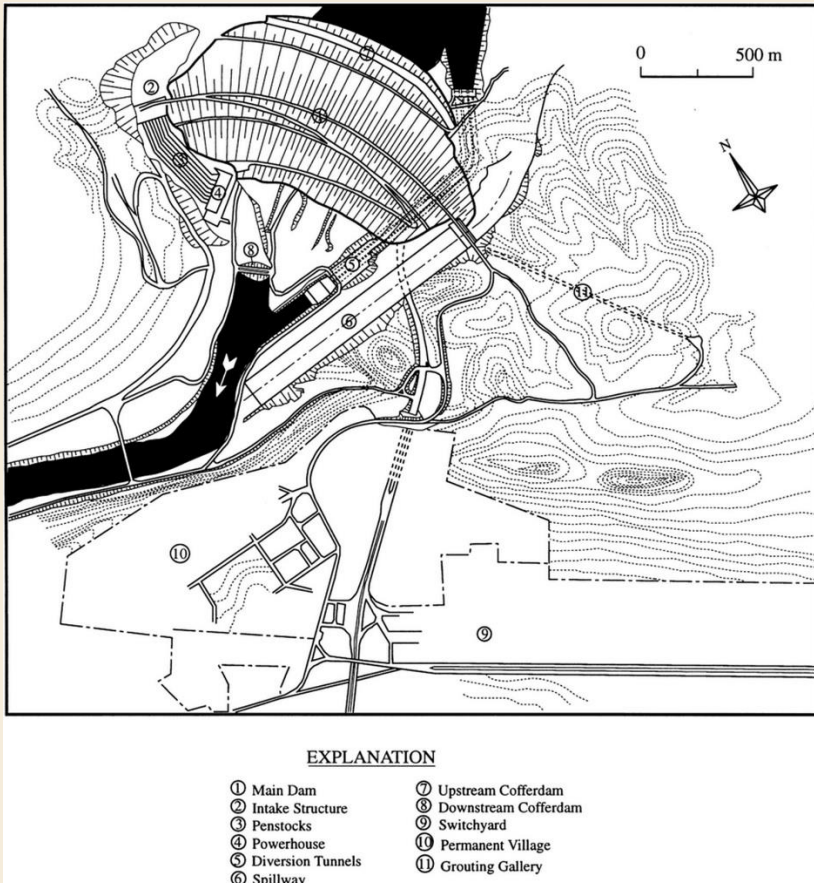
← Az Atatürk-gát üzemi területének áttekintő rajza.
