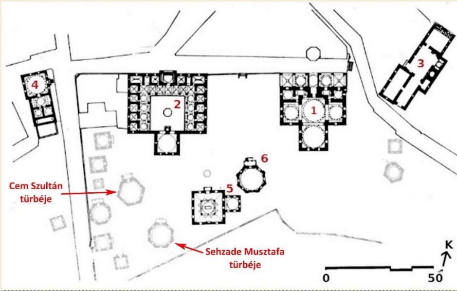
(Resim.2) Bursa Muradiye Külliyesi vaziyet planı (ölçeksiz).
